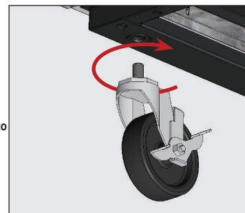
Fig. 8 Avvitare le rotelle orientabili nei fori filettati.
