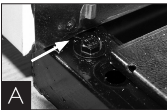
Transportgestell von der Unterseite des Gerätes entfernen
